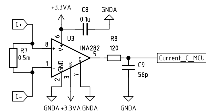
Измерение тока С
