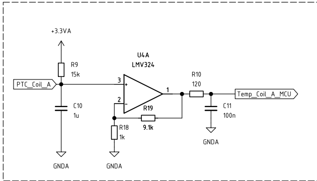
Температура обмотки А
