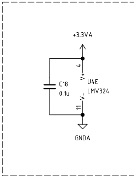
Питание ОУ
