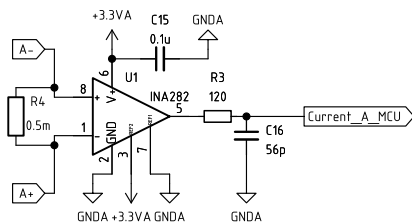
Измерение тока А
