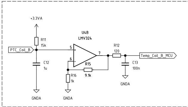
Температура обмотки В
